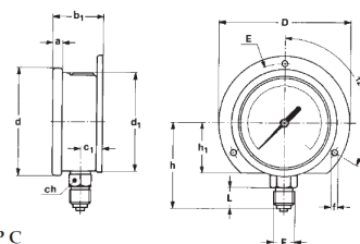
TYP C Fläns i bakkant anslutning nedåt.
