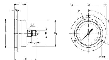
TYP E Panelmontage med frontfläns; anslutning bakåt.
