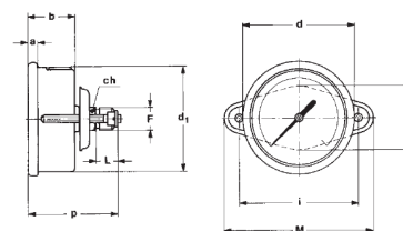
TYP B Panelmontage med bygel; anslutning bakåt
